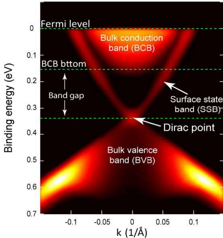
ARPES spectra
